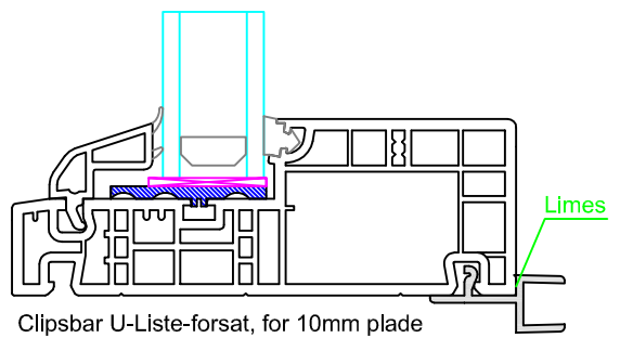
Clipsbar U-Liste-forsat, for 10mm plade Notprofil 2
