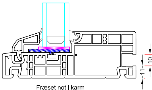
Fræset not i karm
