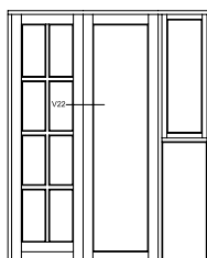
Udadg. pladedør Snit i lodret midtersamling
